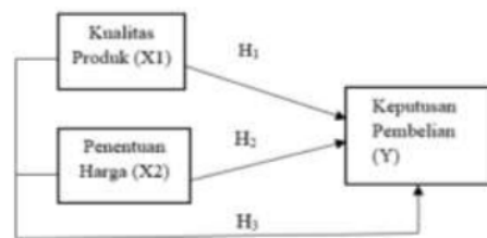
Gambar 2. Kerangka Pemikiran
